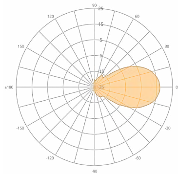
N5-X16 (16 dBi)
